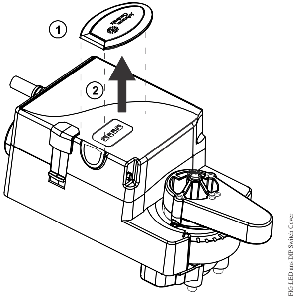
図 13: ディップスイッチと LED のカバー
