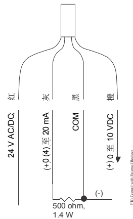
图 12: 比例 24 V 应用 - 0 (4) 至 20 mA (外接电阻)
