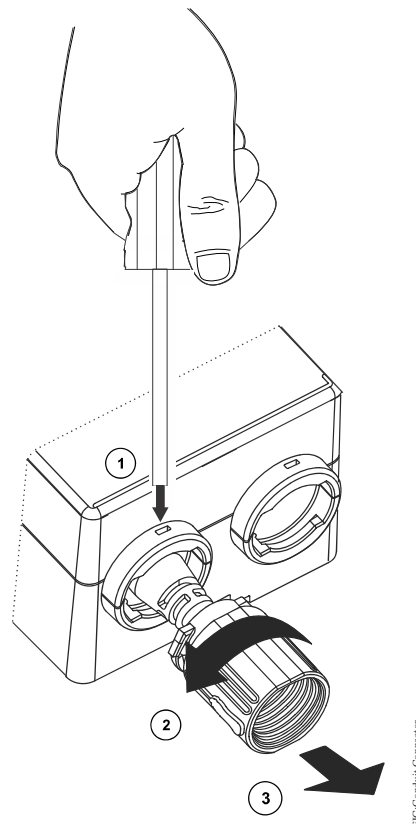
图 17: 拆卸导管连接器
