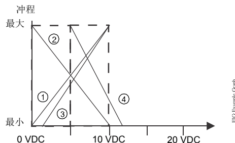
图 15: 表 3 命令信号图示
