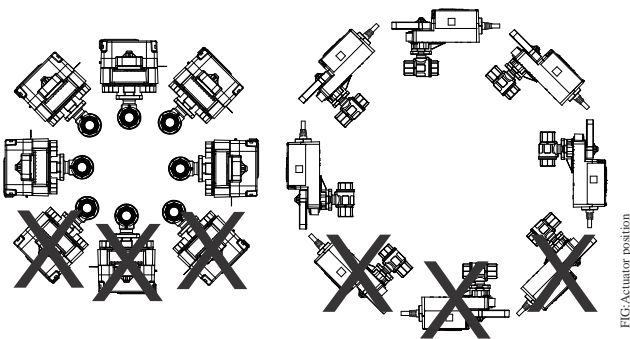
图 2: 安装位置
