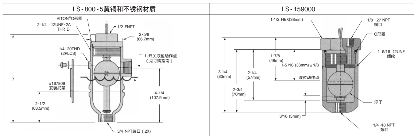
3/4 NPT端口
