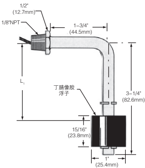
I 型 – 1/8" NPT
